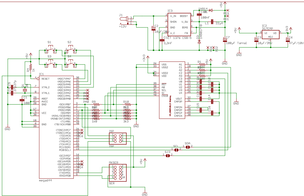
Mobiles Koptertool
